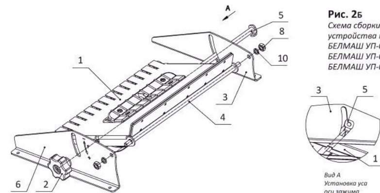
Рис. 2а Схема сборки устройства прижимного БЕЛМАШ УП-2000 БЕЛМАШ УП-2200 БЕЛМАШ УП-2500
